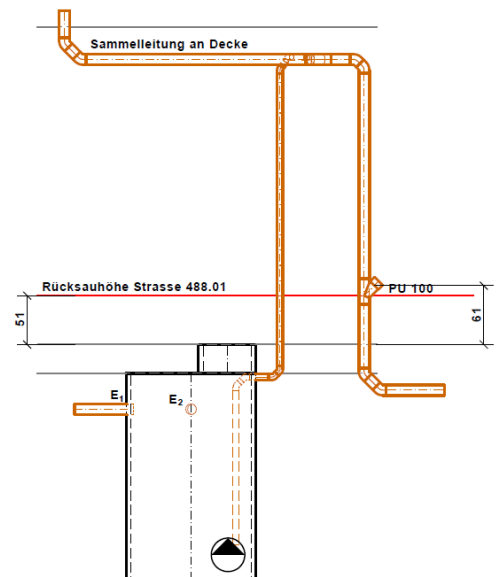
Detail Schmutzwasserpumpe 1:50
